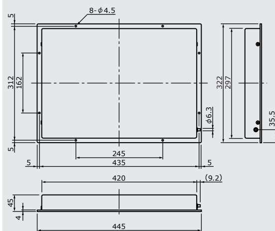
■寸法図 (記載寸法は参考値)
